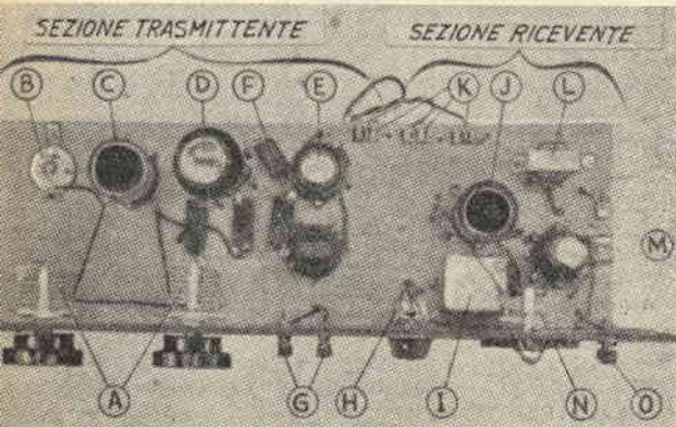
Fig. 3 - Il ricetrasmittitore veduto dall'alto. A) condensatore sintonia trasmettitore; B) Zoccolo lampada sintonia antenna; C) Bobina trasmettitore; D) 6L6G; E) 6J5G; F) Cristallo; G) tasto telegrafico; H) Potenziometro comando reazione; I) Condensatore 1 mf.; J) Bobina ricevitore; K) Terminali alimentatore; L) Trasformatore AF; M) 6CN7; N) 50 mmf. condensatore sintonia ricevitore; O) terminali cuffie.
