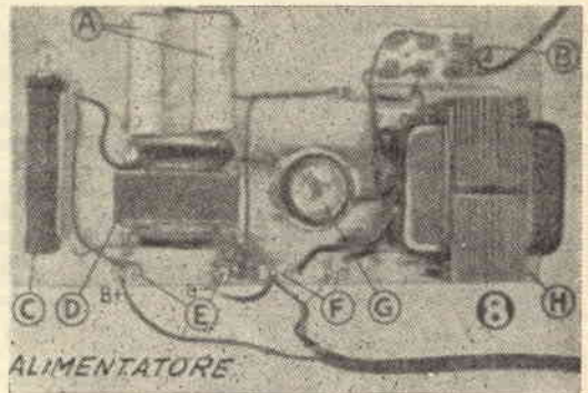
Fig. 8 - L'alimentatore: A) condensatori di filtro; B) interruttore linea alim.; G) resistenza 50 watt; D) impedenza di filtro; E) morsetti per terminali alimentazione; F) 6,3 volts corr. altern.; H) zoccolo raddrizzatrice; H) trasformatore alimentazione.
