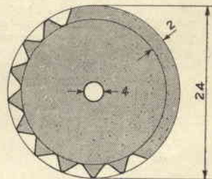
MATER: OTTONE 1,5 ; 18 DENTI
