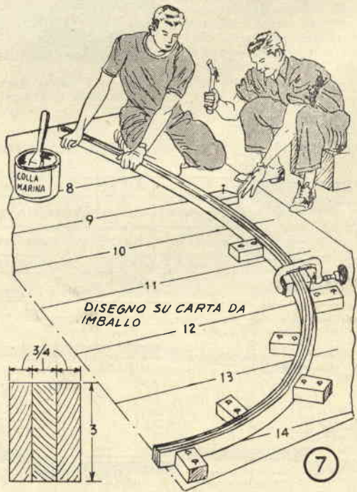
SUPPORTI LAMINATI DEL QUADRATO
